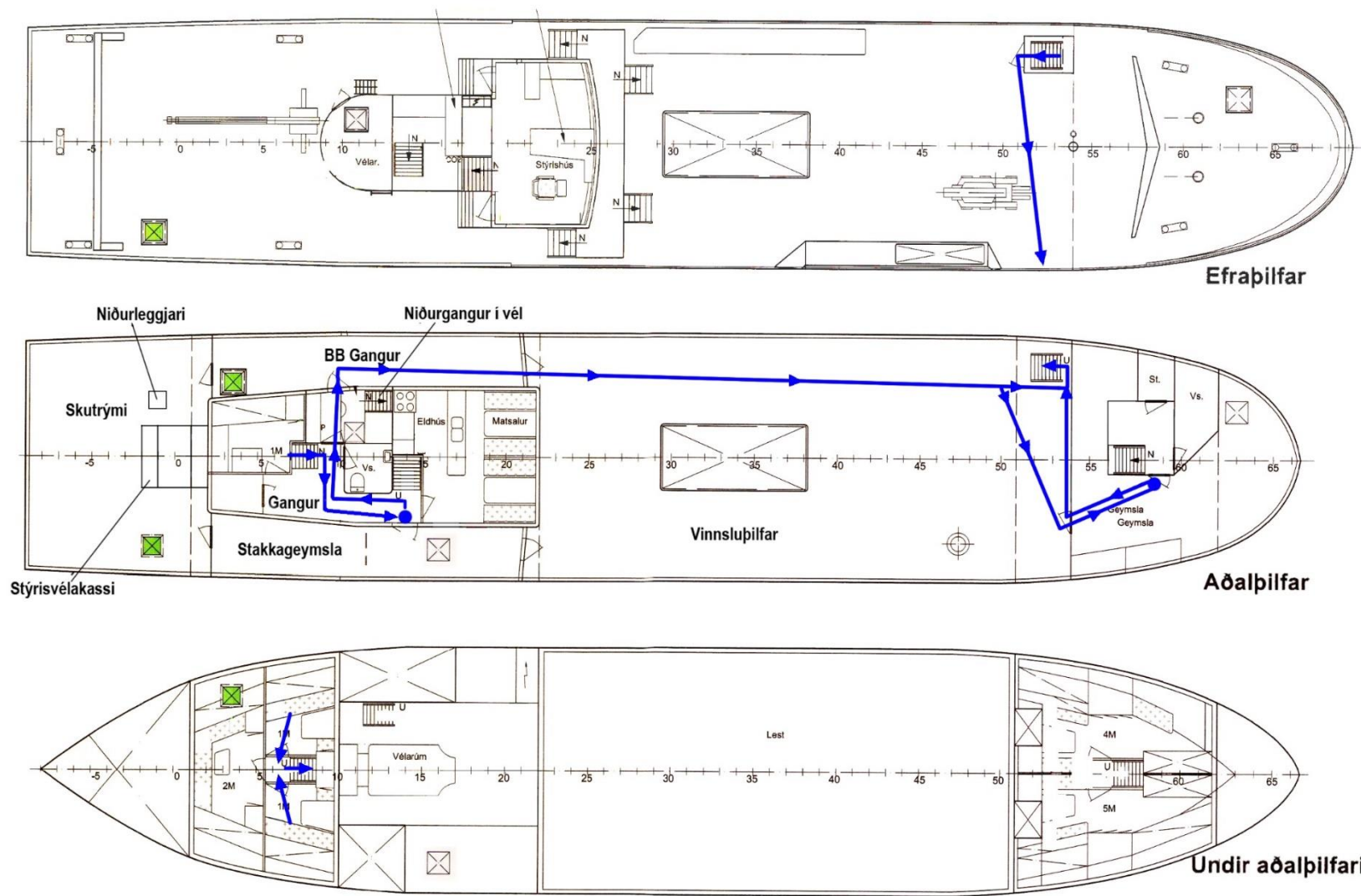
Mynd 2. Sýnir leið þeirra tveggja sem voru í einmenningsklefunum afturí. Eins og fyrr segir fóru þeir upp og út að útgangi í stakkageymslu, til baka út í bakborðsgang og fram eftir vinnsludekkinu. Annar opnaði hurðina upp á efra dekk en hinn vakti þá sem voru frammí og fór síðan upp á efra dekk.
