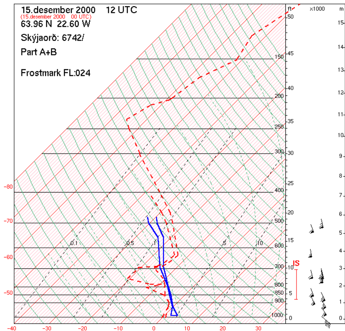
Mynd 5 - Háloftaathugun frá Keflavíkurlugvelli 15. desember 2000 12 UTC. Hiti og daggarmark er táknað með blárri, heilli línu. Síðasta athugun, frá miðnætti aðfaraþótt 15. desember, er sýnd með rauðri stríkalínu.
