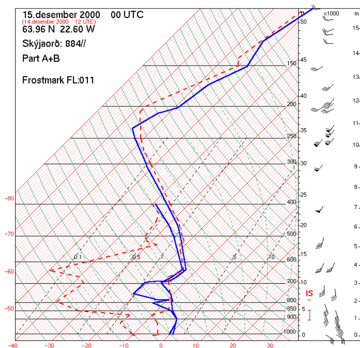
Mynd 4 - Háloftaathugun frá Keflavíkurflugvelli 15. desember 2000 00 UTC. Hiti og daggar-mark er táknað með blárri, heilli línu. Síðasta athugun, frá hádegi þann 14. desember, er sýnd með rauðri strikallínu.
